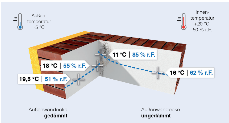
03 Absenkung der Temperatur und Anstieg der relativen Luftfeuchte einer gedämmten und einer ungedämmten Außenwanddecke. Schematische Darstellung zu Anschauungszwecken.
