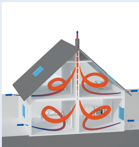
06 Zentrale Abluftanlage
