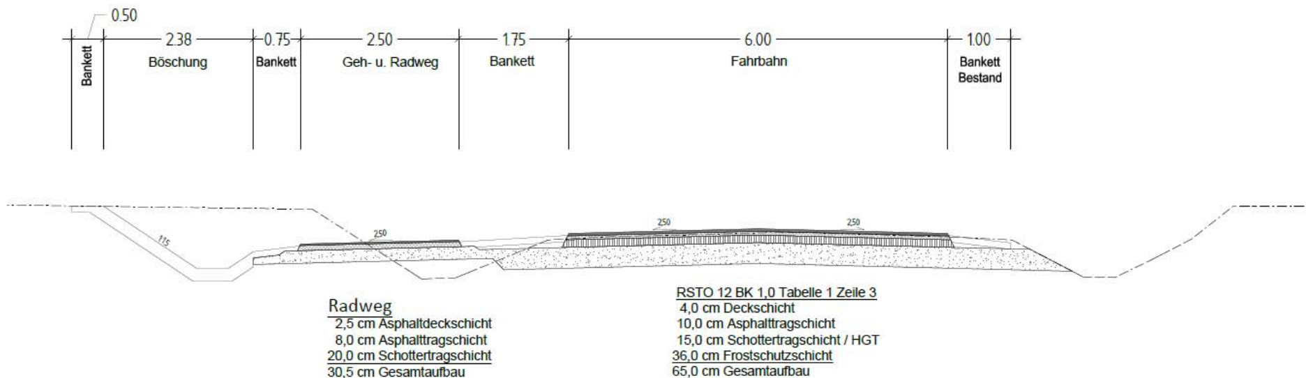
Querschnitt A-A Achse 200 Station 0+170
