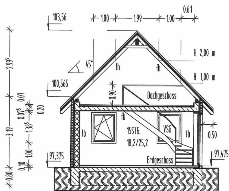
Schnitt A
